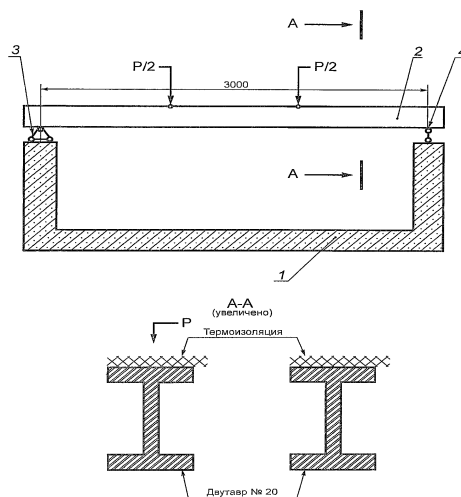
1 - огневая камера печи; 2 - опытный образец стальной балки; 3 - шарнирно-неподвижная опора; 4 - шарнирно-подвижная опора
