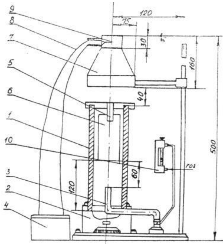
Рис. 1. Установка для определения огнезащитной эффективности ОЗСВ:
